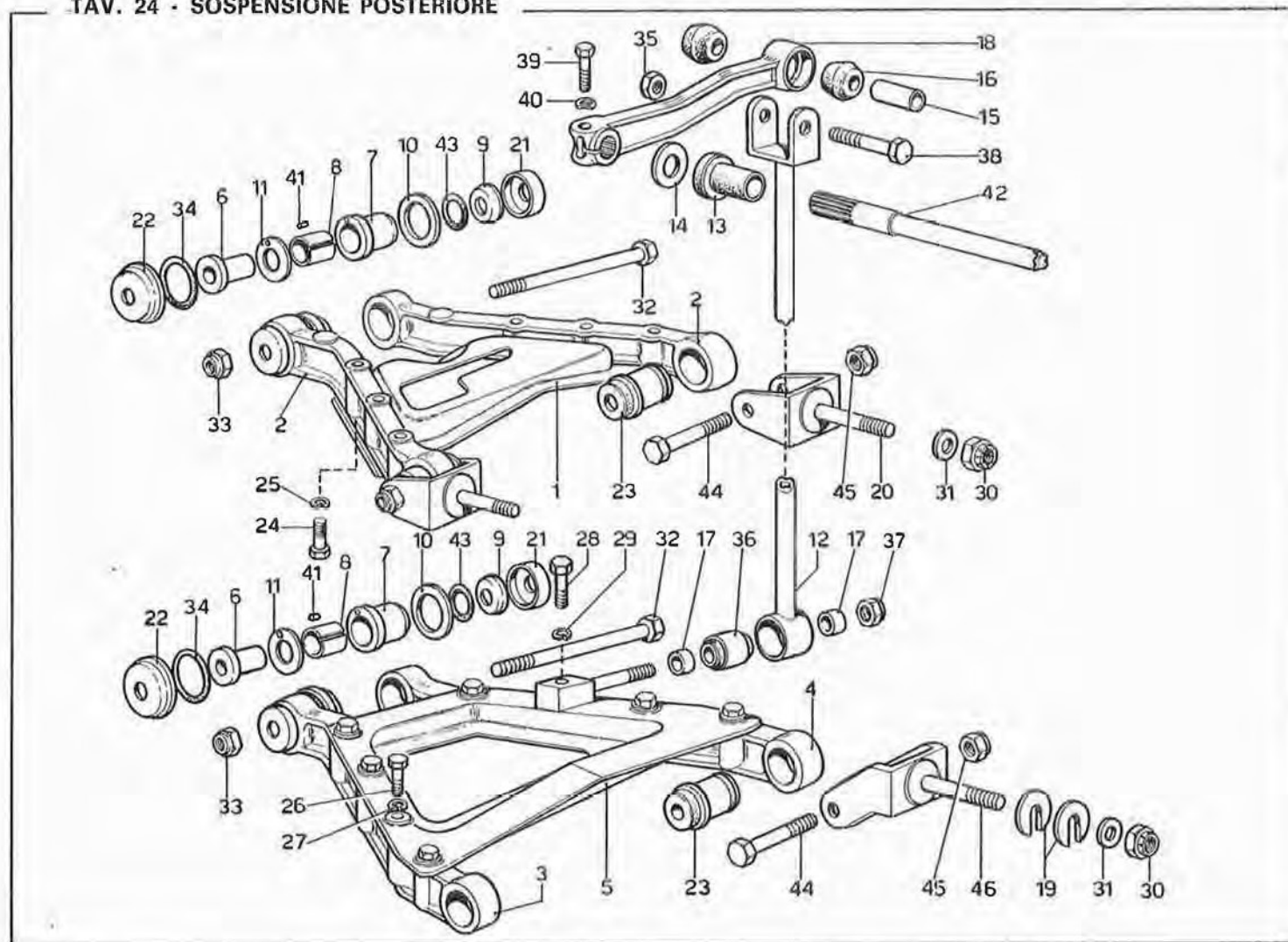
TAV. 24 - SOSPENSIONE POSTERIORE
