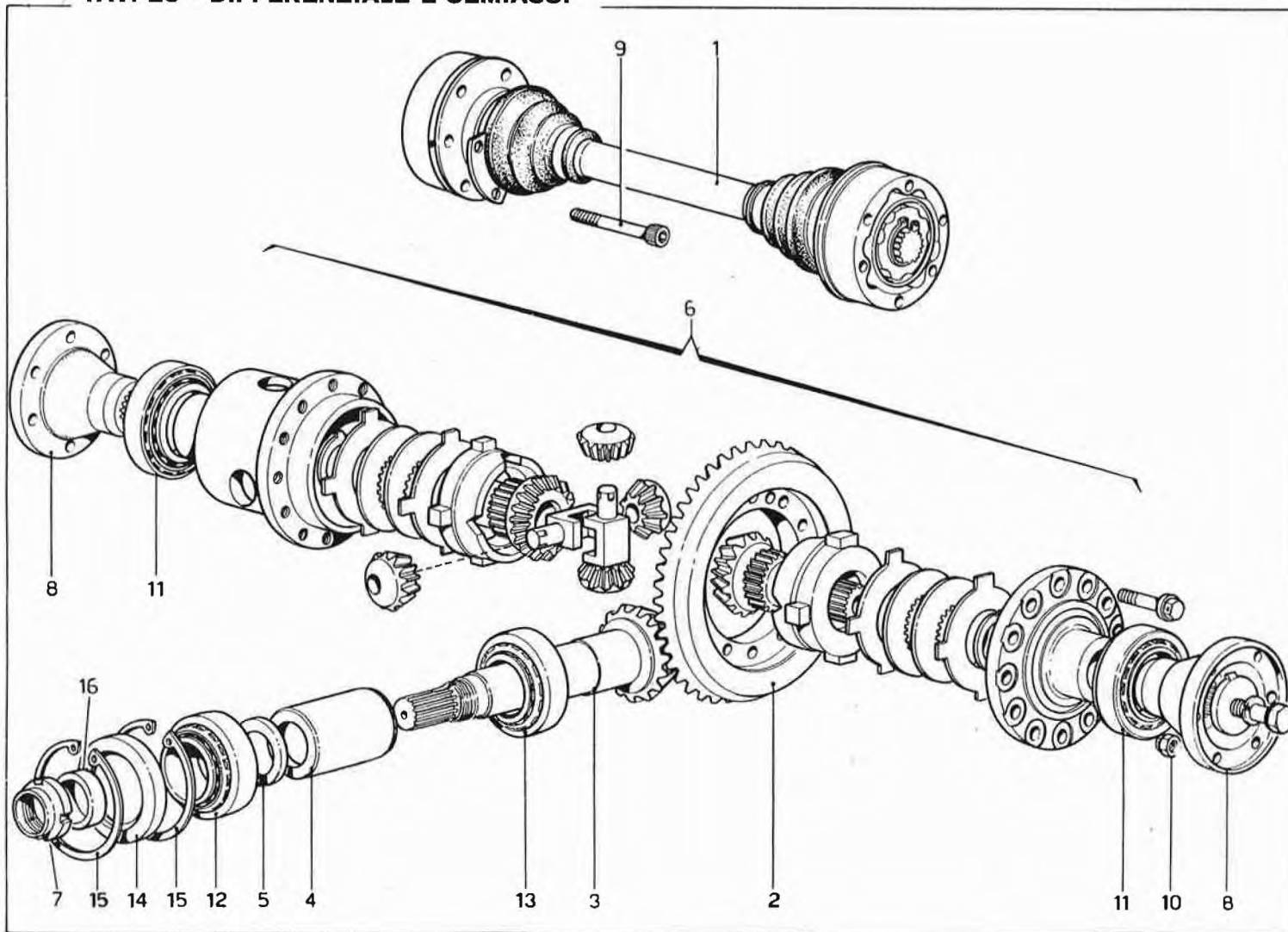
TAV. 28 - DIFFERENZIALE E SEMIASSI
