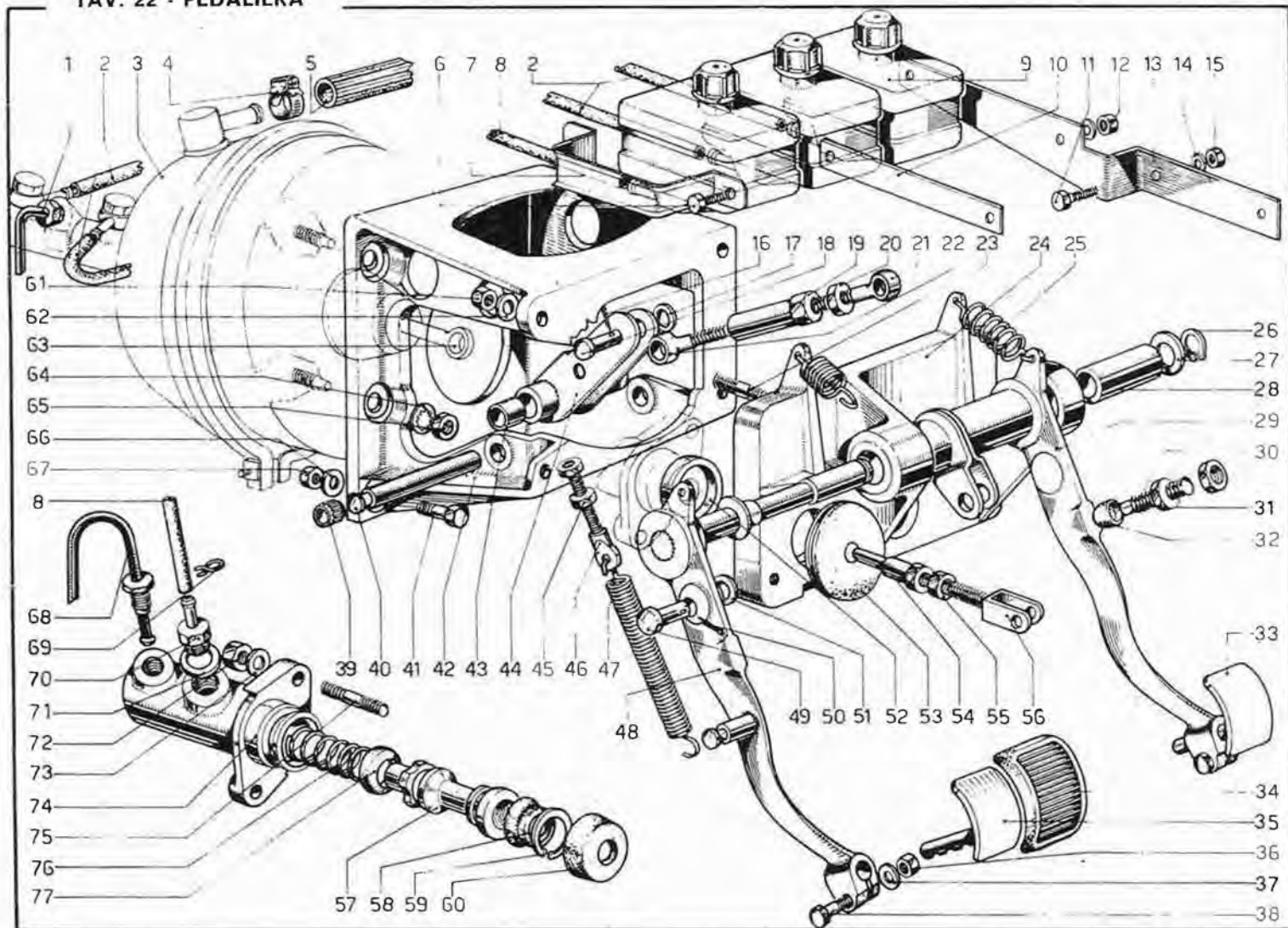
TAV. 22 - PEDALIERA
