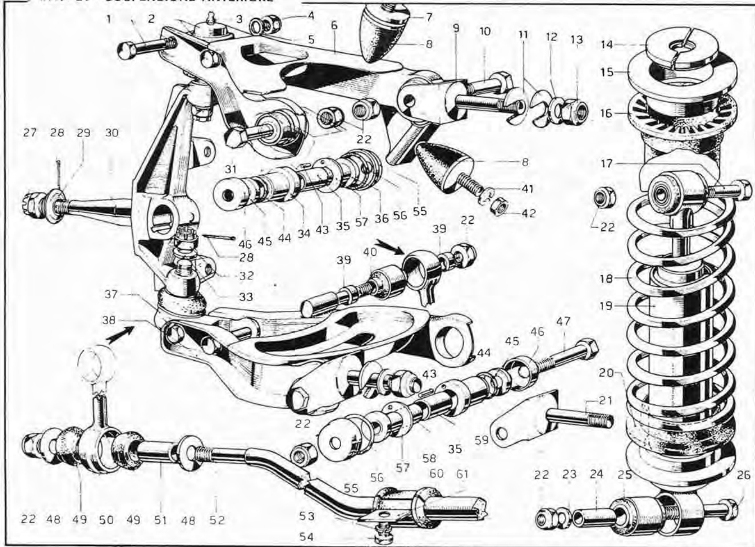
TAV. 21 - SOSPENSIONE ANTERIORE
