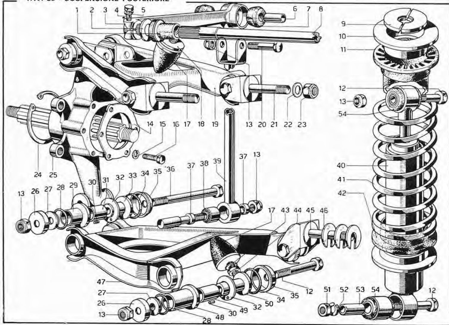
TAV. 20 - SOSPENSIONE POSTERIORE
