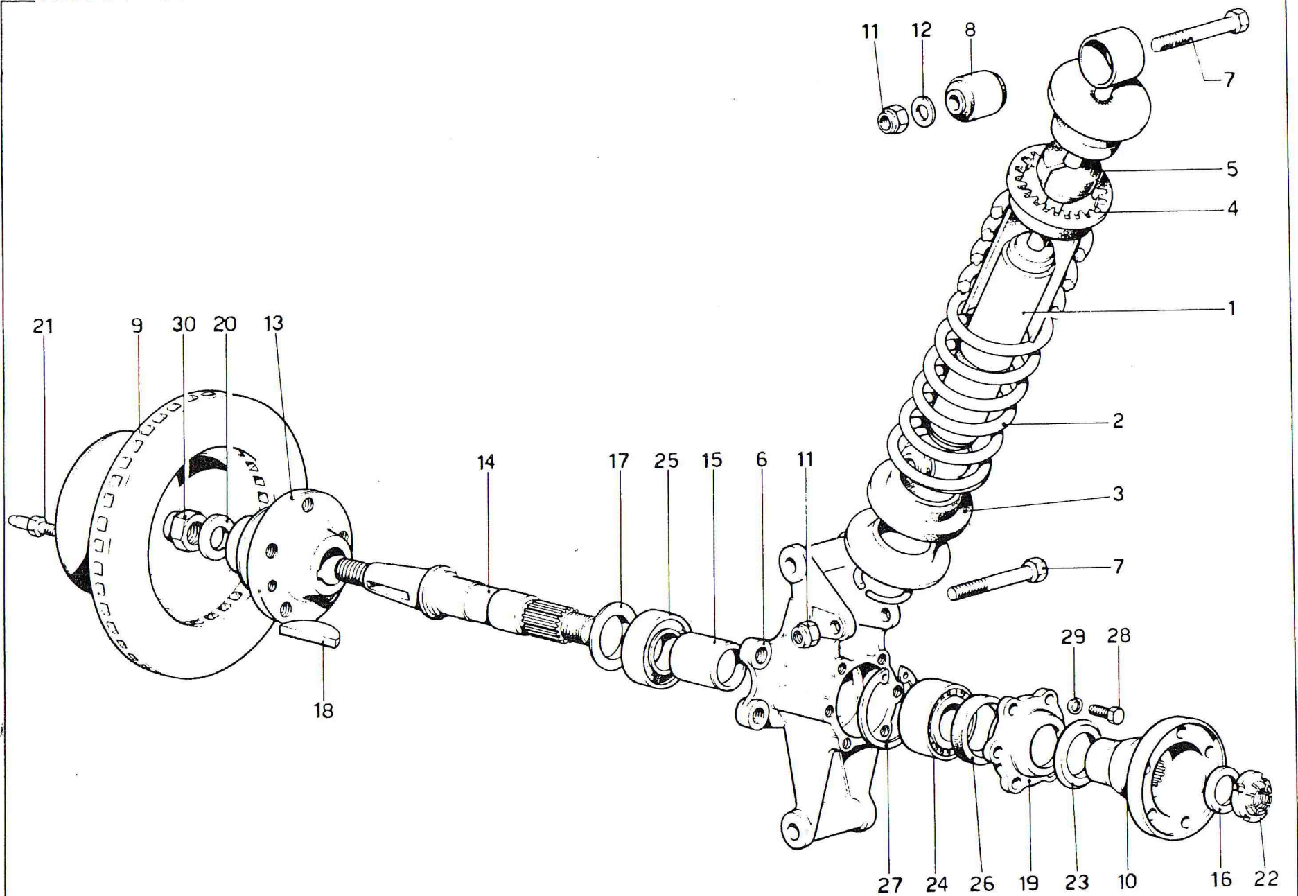
TAV. 34 - SOSPENSIONE POSTERIORE - AMMORTIZZATORE
