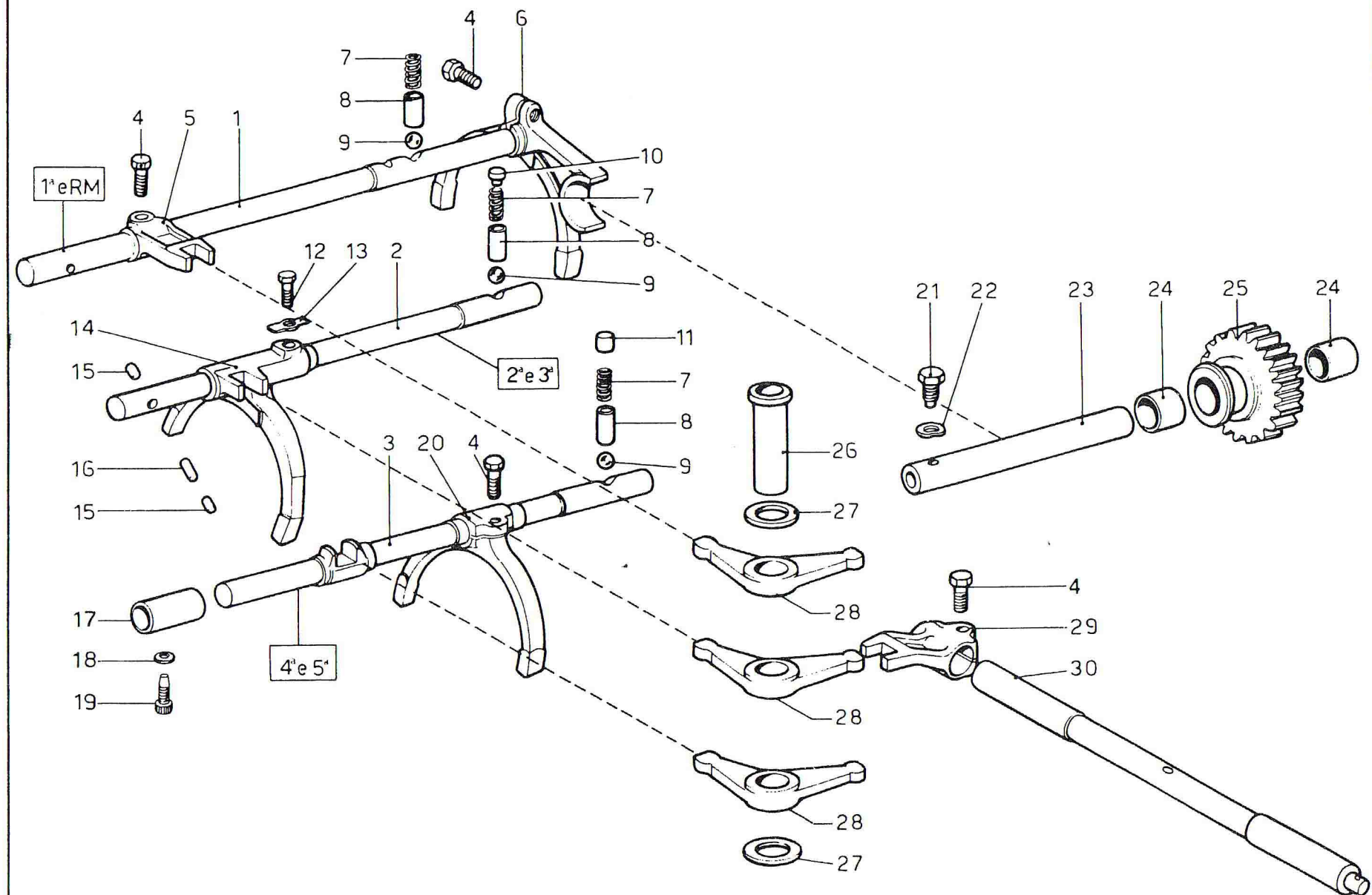
TAV. 24 - COMANDI INTERNO CAMBIO
