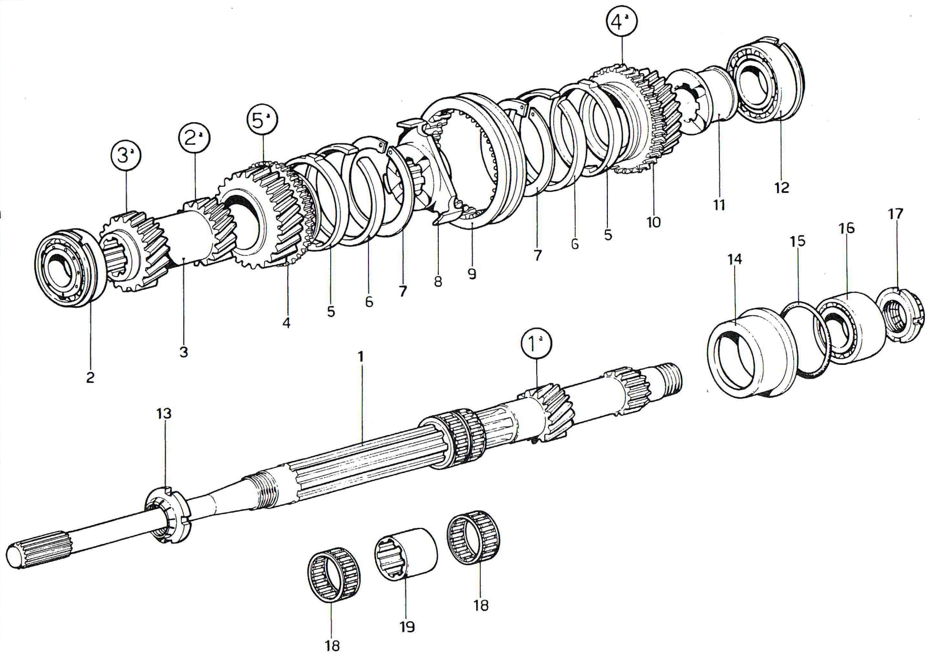
TAV. 21 - RUOTISMI ALBERO PRIMARIO CAMBIO
