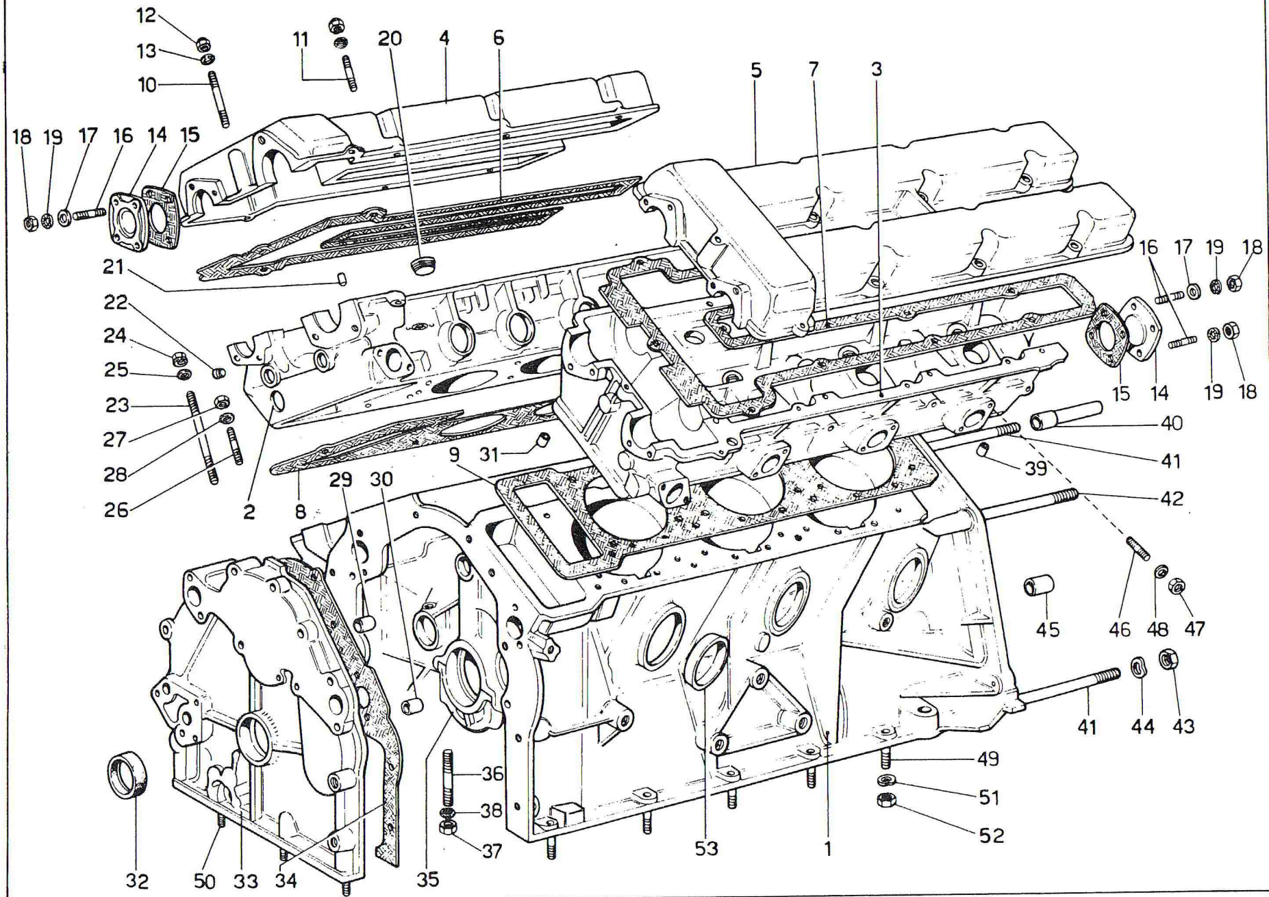
TAV. 1 - BASAMENTO E TESTE CILINDRI
