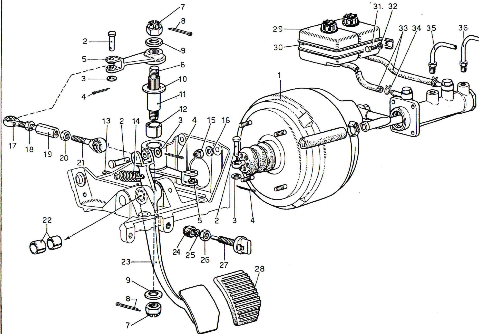
TAV. 26 - COMANDO IDRAULICO FRENI
