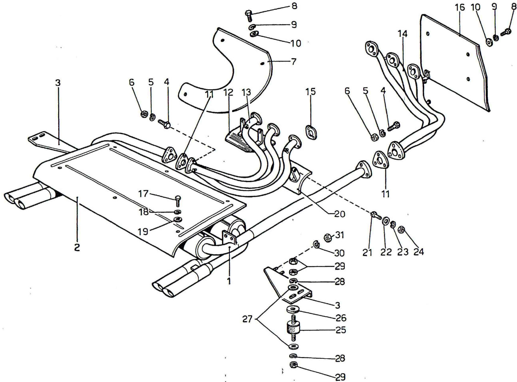
TAV. 13 - IMPIANTO SCARICO
